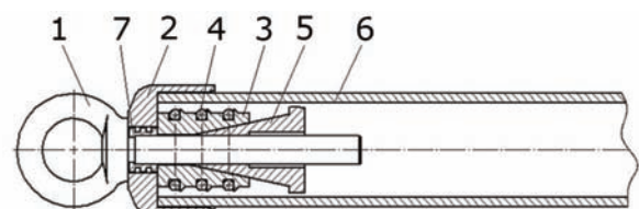
Ziehkopf mit Abdichtung
