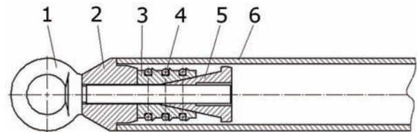
Ziehkopf ohne Abdichtung
